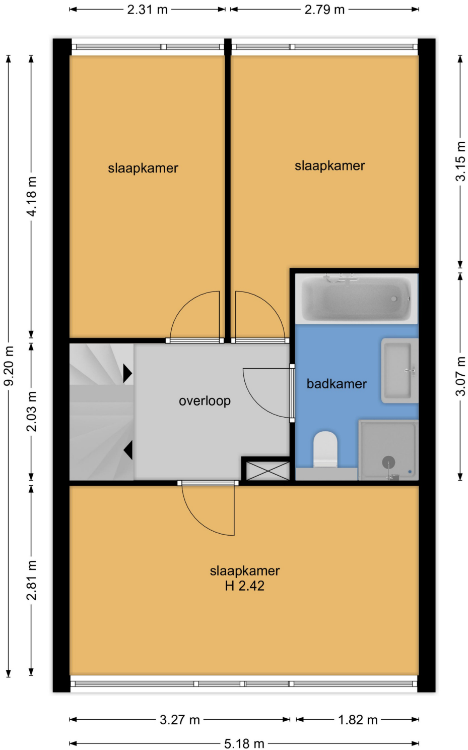
1e verdieping
